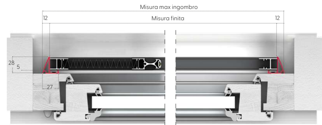
Plissè 22 fissaggio fronte tondo
